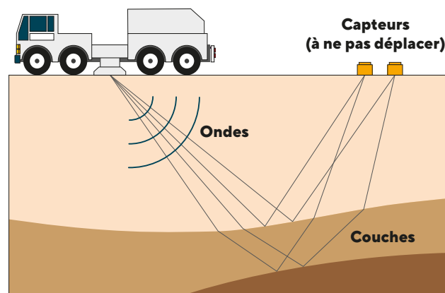
Camion-vibreur Thomas T65 ©S3
